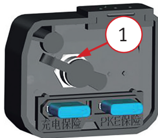
Фото 4.1 Место подключения зарядки АКБ: 1 – розетка для зарядки.
