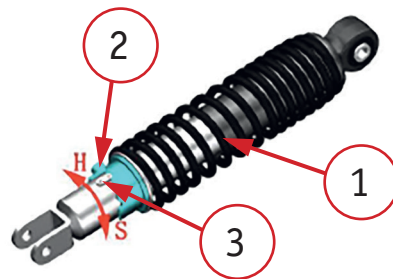
Фото 2.20. Регулировка преднатяга амортизатора: 1 – пружина; 2 – регулятор; 3 – фиксатор. «S» - направление вращения для ослабления преднатяга; «Н» - направление вращения для увеличения преднатяга.
