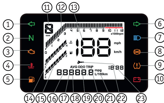
Фото 2.8. Приборная панель моделей ZT125-U/U1, ZT200-U1, ZT125-Z2: 1 - индикатор левого поворота; 2 - индикатор нейтральной передачи; 3 - индикатор неисправности двигателя; 4 - индикатор температуры охлаждающей жидкости; 5 - индикатор низкого уровня топлива; 6 - индикатор правого поворота; 7 - индикатор дальнего света; 8 - индикатор системы ABS; 9 - индикатор низкого давления в шинах; 10 - индикатор низкого напряжения аккумулятора; 11 - текущая передача; 12 - тахометр; 13 - спидометр; 14 - шкала температуры охлаждающей жидкости; 15 - шкала уровня топлива; 16 - давление в передней/задней шине; 17 - запас хода на оставшемся топливе; 18 - средняя скорость; 19 - общий километраж; 20 - текущий километраж; 21 - расход топлива; 22 - часы/коды неисправности давления в шинах; 23 - индикатор необходимости проведения ТО.
