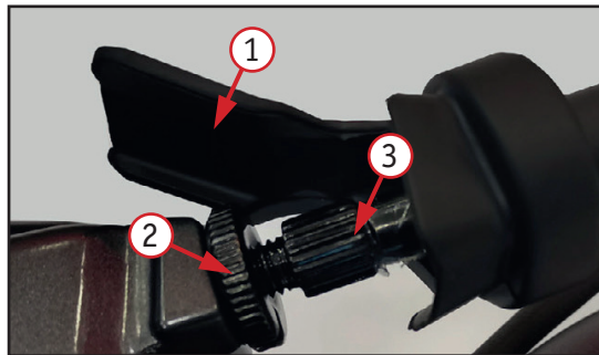
Рисунок 1. Свободный ход рычага сцепления.
