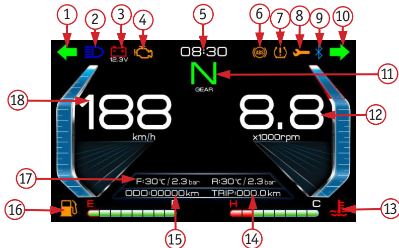
Фото 2.7. Приборная панель: 1 – индикатор левого поворота; 2 – индикатор дальнего света; 3 – индикатор напряжения аккумулятора; 4 – индикатор неисправности двигателя; 5 – часы; 6 – индикатор системы ABS; 7 – индикатор низкого давления в шинах; 8 – индикатор ТО; 9 – индикатор Bluetooth-подключения; 10 – индикатор правого поворота; 11 – текущая передача; 12 – тахометр; 13 – шкала температуры охлаждающей жидкости; 14 – текущий километраж; 15 – общий километраж; 16 – шкала уровня топлива; 17 – температура воздуха/давление в шинах; 18 – спидометр
